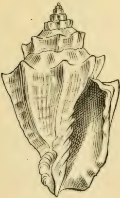
Fig. 271.
